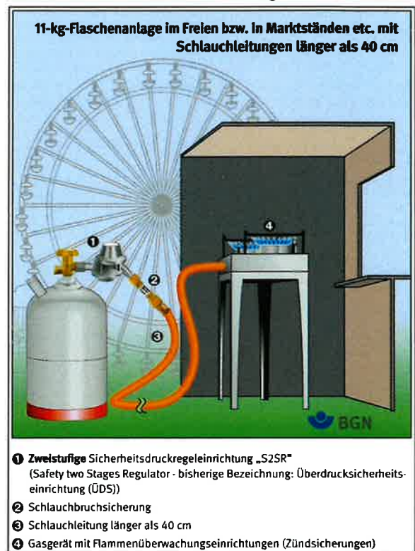
Bild 1 Beispielhafte Flüssiggasanlage
